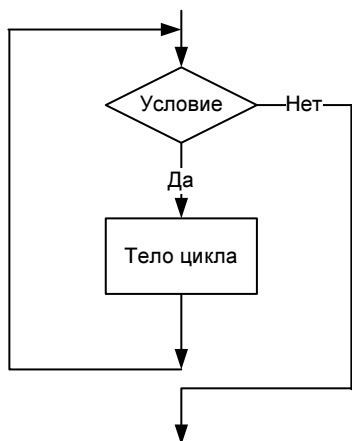
Рис. 1.5. Цикл с предусловием
