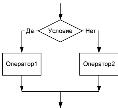
Рис. 1.3. Полная развилка
