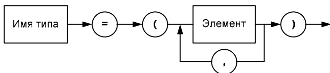
Рис. 2.4. Синтаксическая диаграмма перечислимого типа
