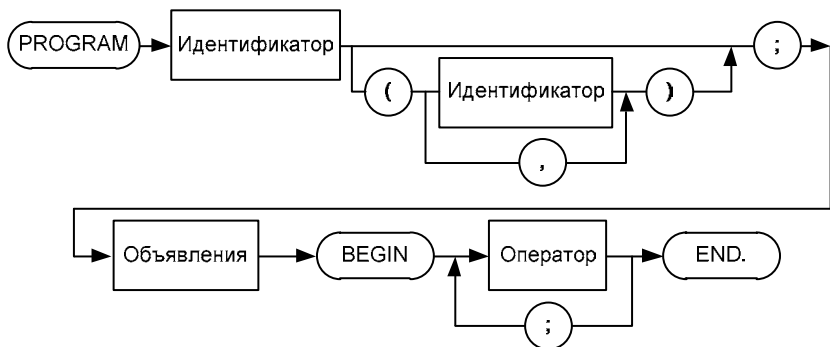
Рис. 2.2. Синтаксическая диаграмма паскаль-программы
