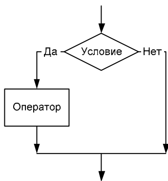
Рис. 1.4. Неполная развилка
