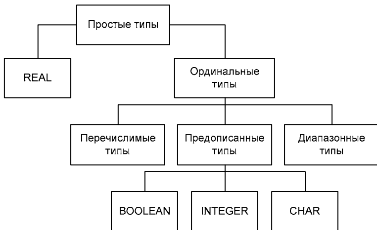
Рис. 2.3. Типизация данных
