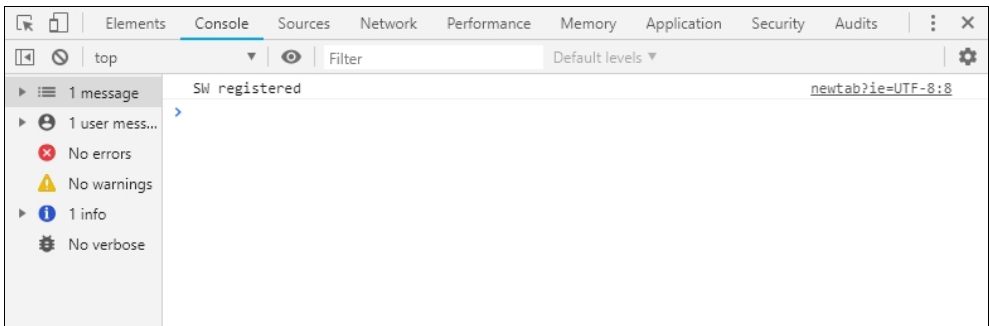
Рис. 1.3. Консоль веб-обозревателя
