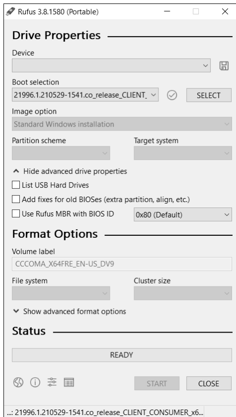
Рис. 1.1. Утилита Rufus
